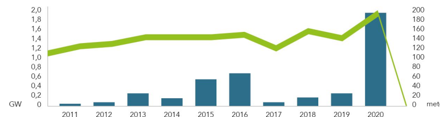
Grafiek (windstats.nl): de groene lijn toont de stijging van de gemiddelde tiphoogte van 100 meter (2010) naar 190 meter (2020). In blauw het jaarlijks opgesteld vermogen in deze tijdreeks met een piek in 2020.
